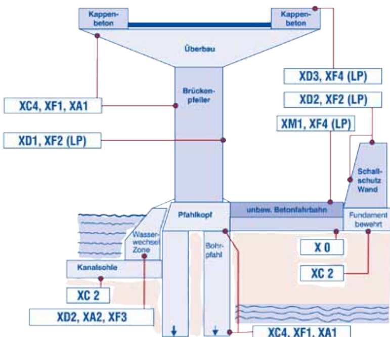
Beispiele für Beton im Industriebau. Für die richtige Auswahl der Betonsorte, ist allein der Abnehmer verantwortlich.
